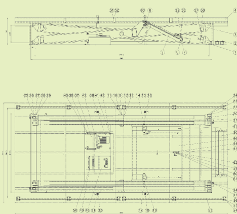
Scherenhubtisch Goliath
