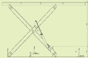
Scherenhubtisch Goliath
